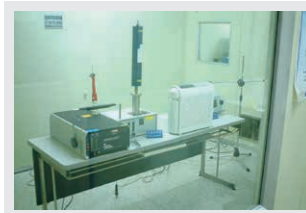
空氣清淨機能源效率測試服務 ANSI/AHAM CADR Test Room
